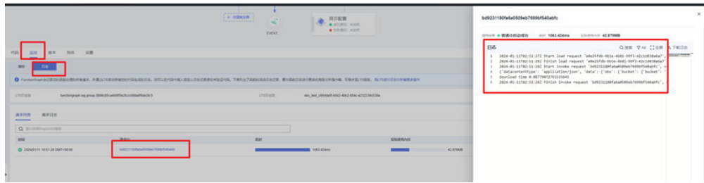
图 3-10 代码日志
