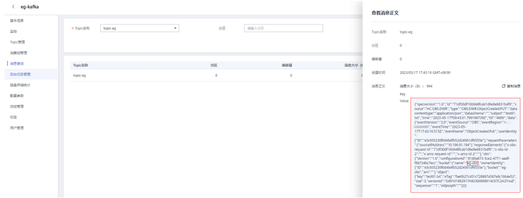
图 1-4 事件消息
