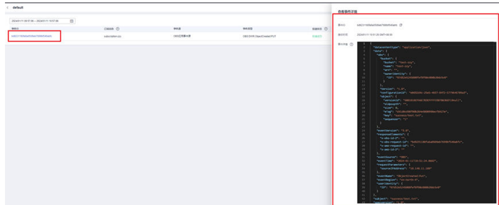
图 3-7 事件详情
